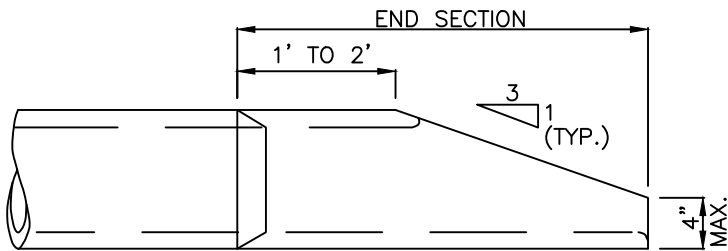
ELEVATION
