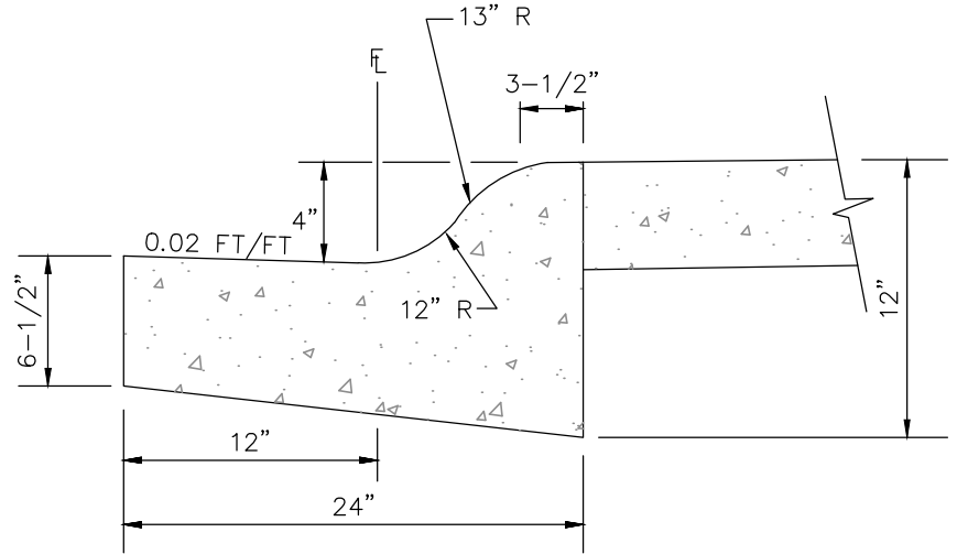
ELEVATION B-B
